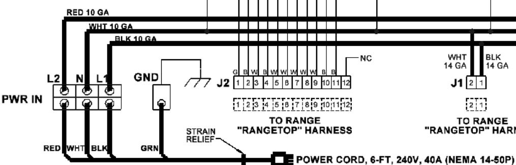
WIRING DIAGRAM, KRD364GD 026234
