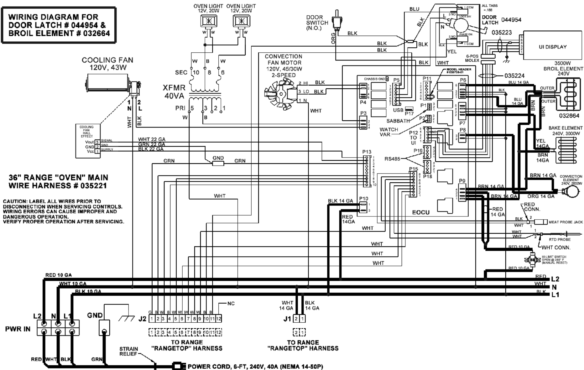
WIRING DIAGRAM, KRD364GD 026234
