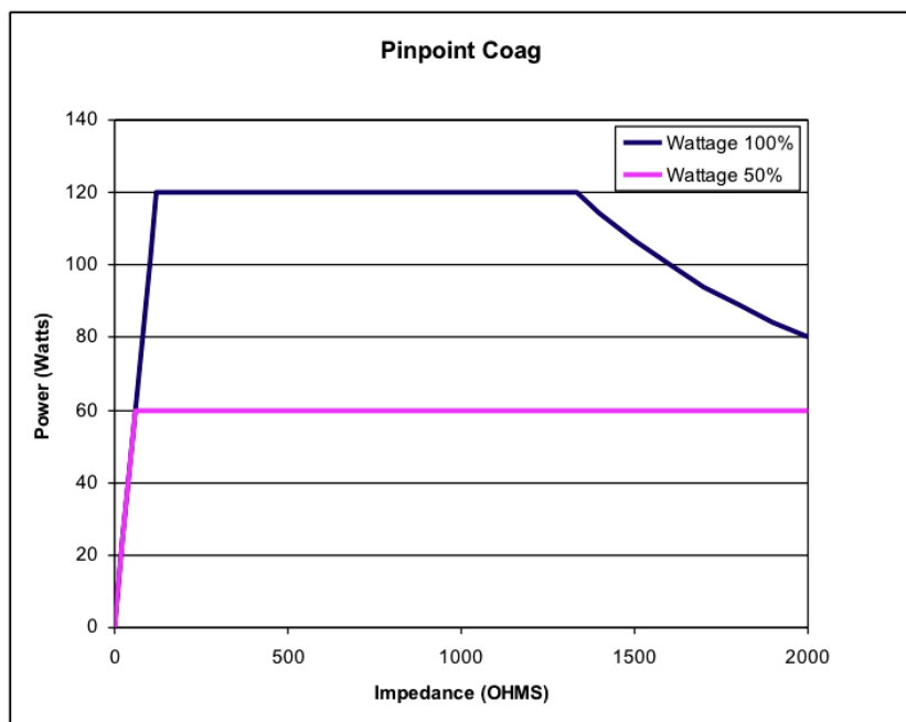
Figura A – 4 Nivelul puterii de ieșire față de impedanță pentru regim PINPOINT COAGULATION
