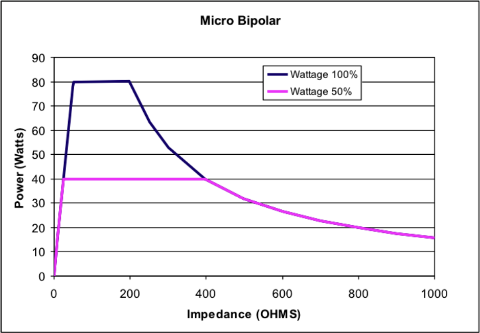
Figura A – 8 Nivelul puterii de ieşire faţă de impedanţă pentru regim MICRO BIPOLAR
