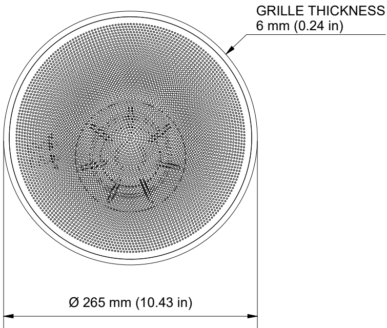
GRILLE
