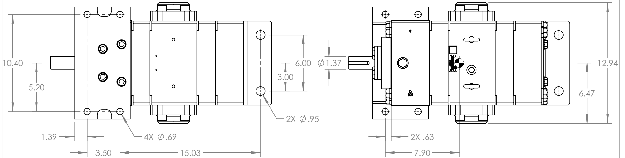
VIEW A-A
