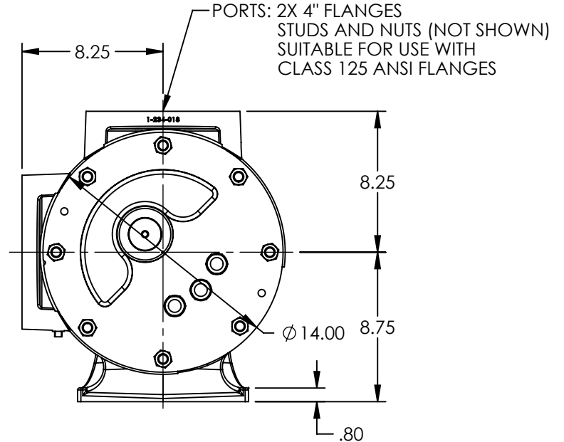
VIEW A-A
