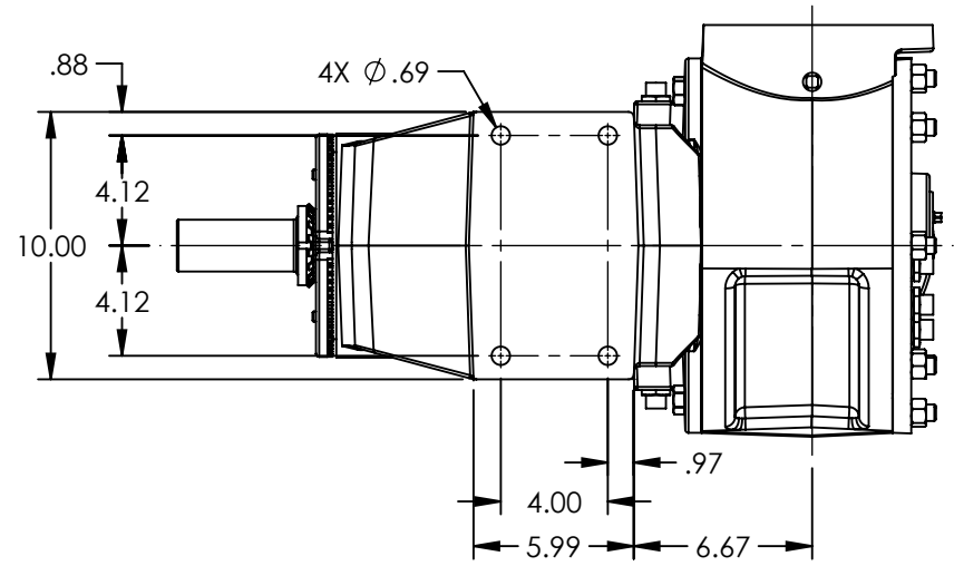
VIEW A-A
