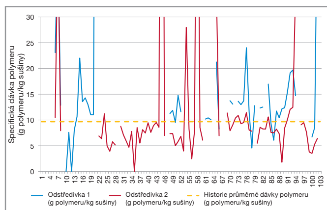
Obrázek 2: Graf vlevo, před optimalizací: Velmi významné kolísání velikosti dávky polymeru vedoucí k nevyhovující kvalitě odvodněného kalu (nedostatečné dávkování) a nutnost použití odpěňovače kvůli nadměrnému dávkování. Graf vpravo, po optimalizaci: Velmi stabilní velikost dávky polymeru – průměrně 5,2 g polymeru/kg sušiny.
