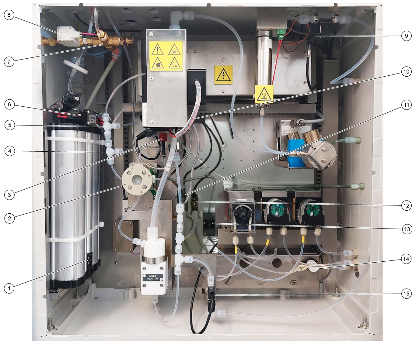
Figur 20 Analyskapsling – Ventiler
