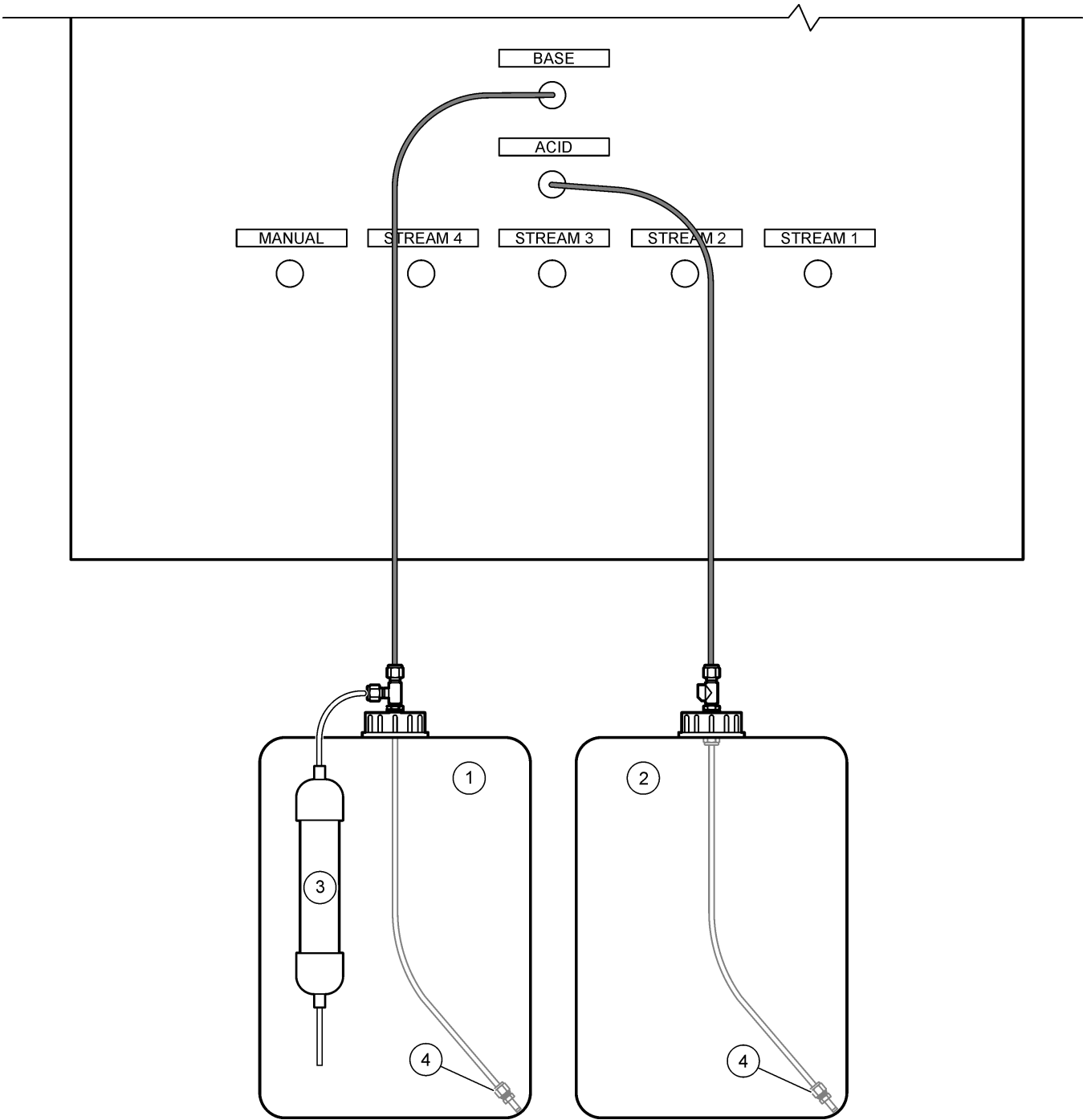
Figura 15 Instalação do reagente
