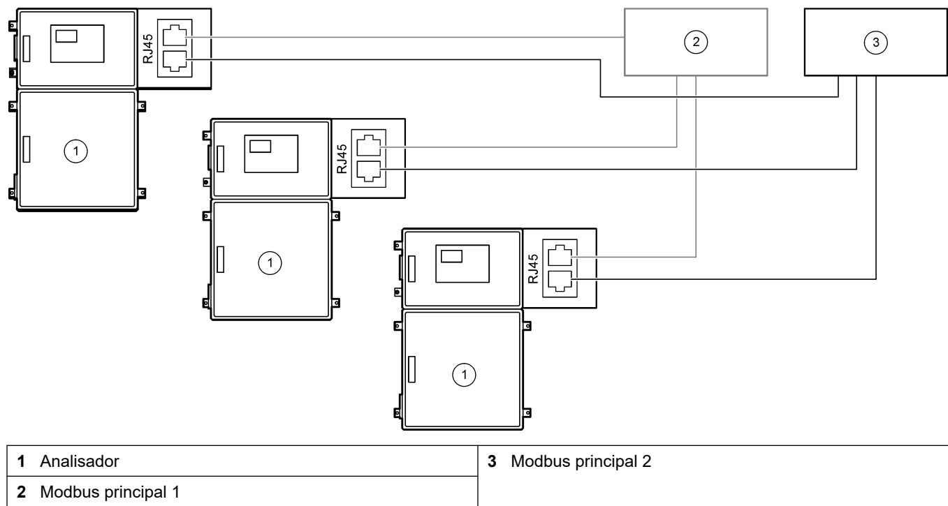
Figura 9 Cablagem do Modbus TCP redundante
