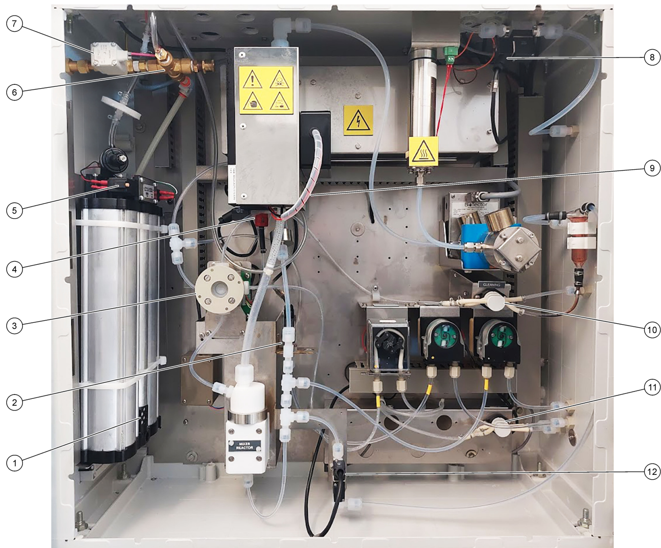
Figura 20 Compartimento de análise – Válvulas
