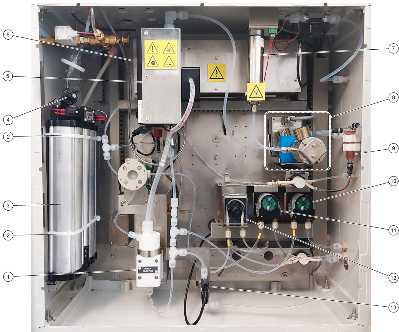
Figura 19 Compartmento de análise – Bombas e componentes
