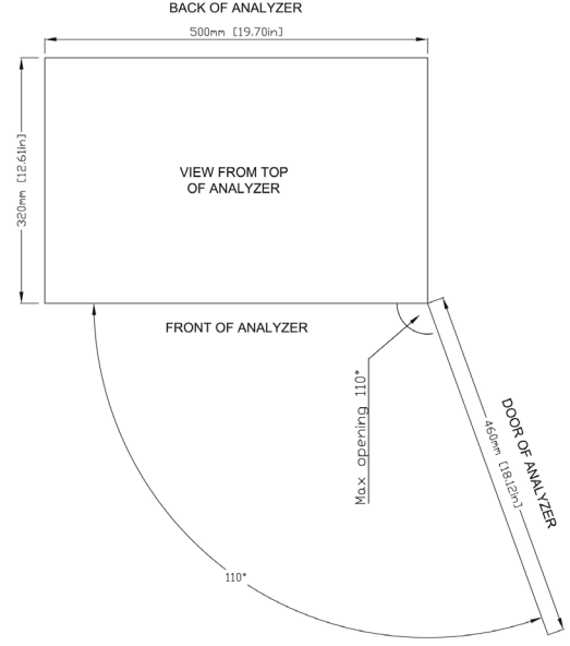
Üstten Görünüm
