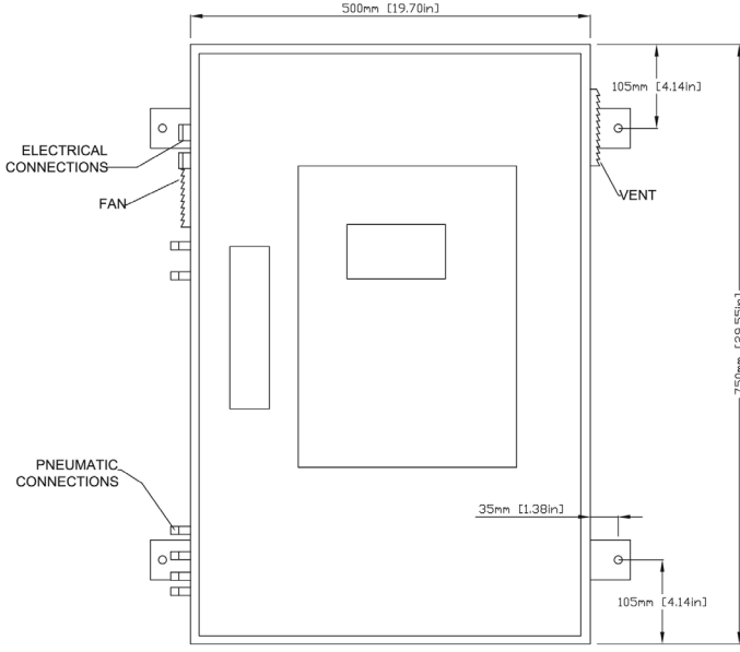
Önden Görünüm
