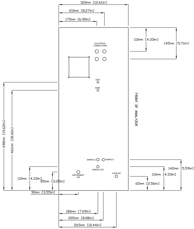
Yandan Görünüm
